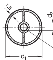
Конструкция для d_1 = 20 и 28
