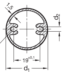
Конструкция для d_1 = 30
