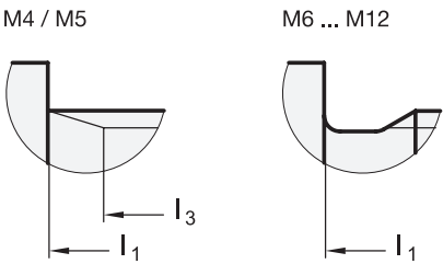
Деталь Z; Сбег резьбы:
