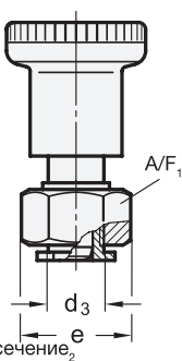
Плунжерный штифт втянут
