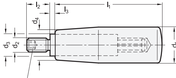
Внутренний шестигранник
