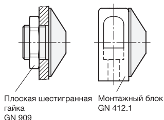
Примеры сборки
