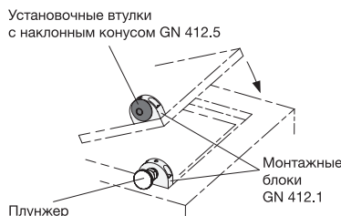
Пример использования
