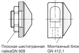
Варианты сборки
