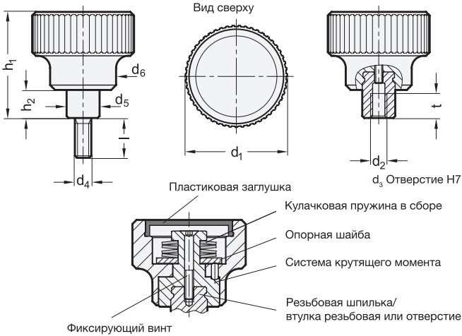
GN 3663-со шпилькой
